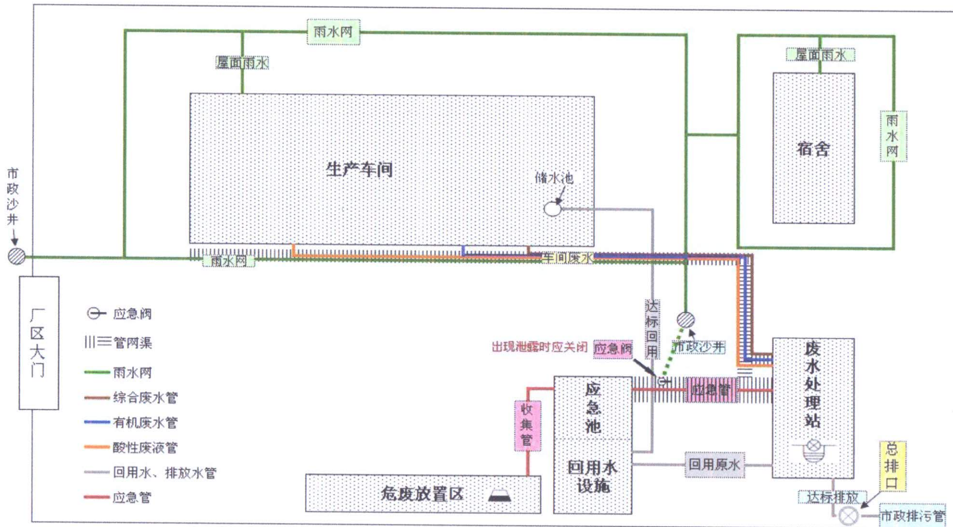
附图 4：雨水、污水流向图
